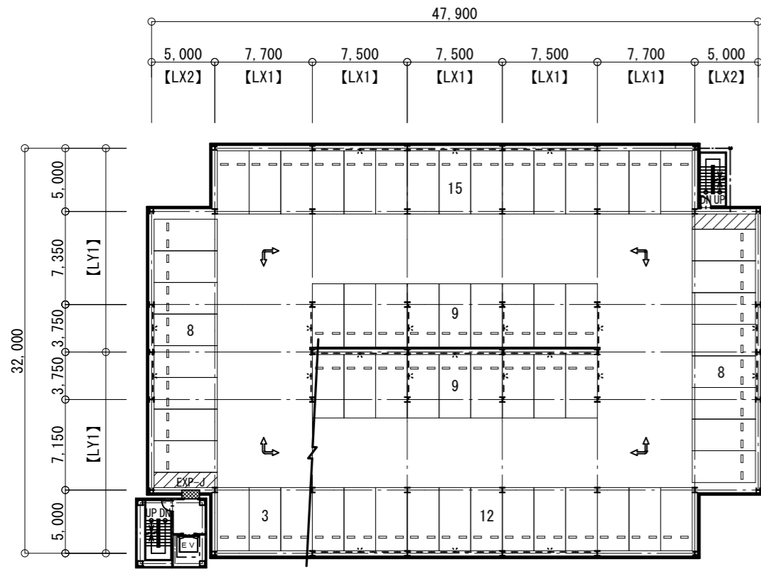
2～6階 平面図
