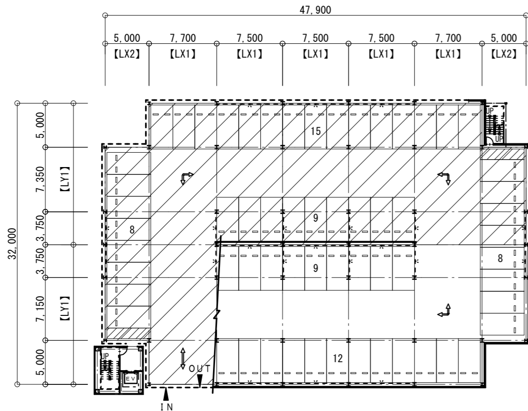
1階 平面図
